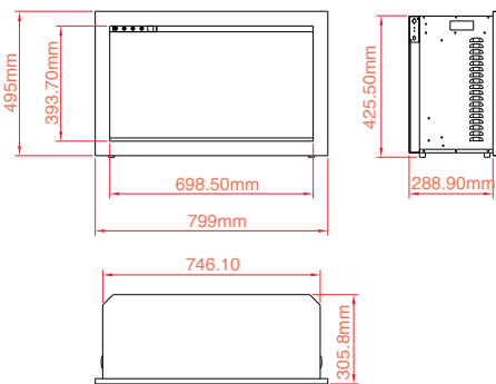
CLASSIC-30
